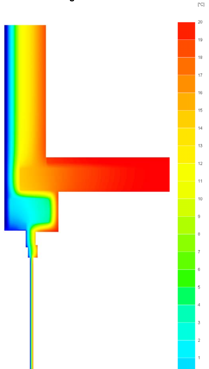
Bild 6 : Einbaudetail B.31
