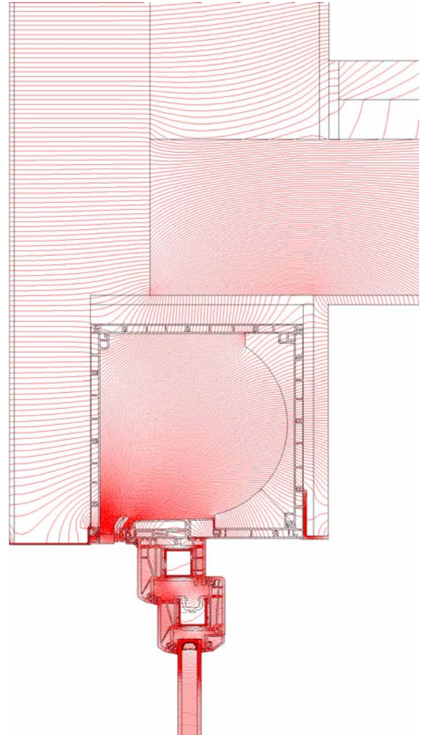
Bild 8 : Einbaudetail
