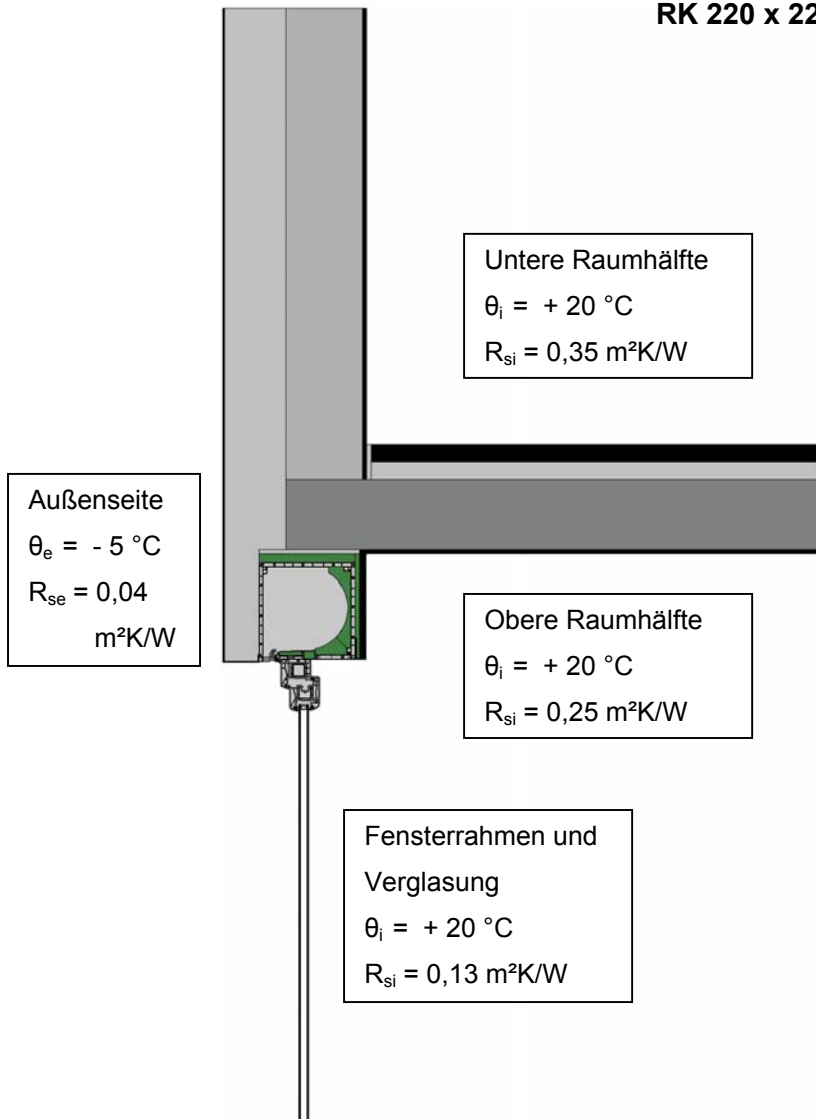
Bild 7 : Einbaudetail mit EXTE Expert RK 220 x 220 Aufbereitung von Bild 1
