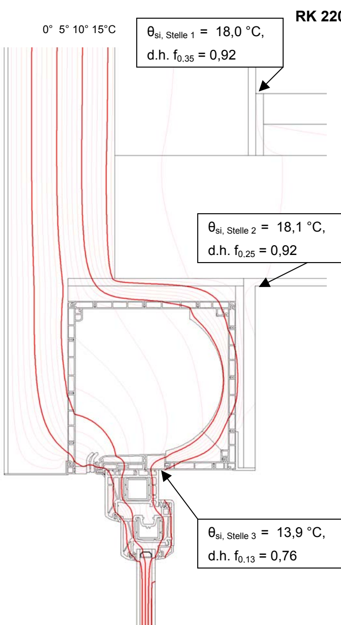
Bild 9 : Einbaudetail mit EXTE Expert RK 220 x 220 (Ausschnitt zur besseren Sichtbarkeit des RK- Bereiches)
