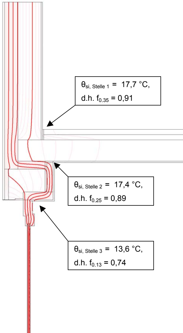
Bild 5 : Einbaudetail B.31
