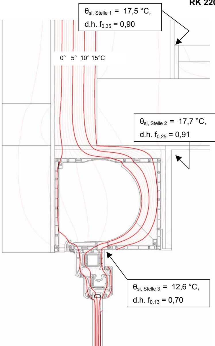
Bild 9 : Einbaudetail mit EXTE Expert RK 220 x 255 (Ausschnitt zur besseren Sichtbarkeit des RK- Bereiches)
