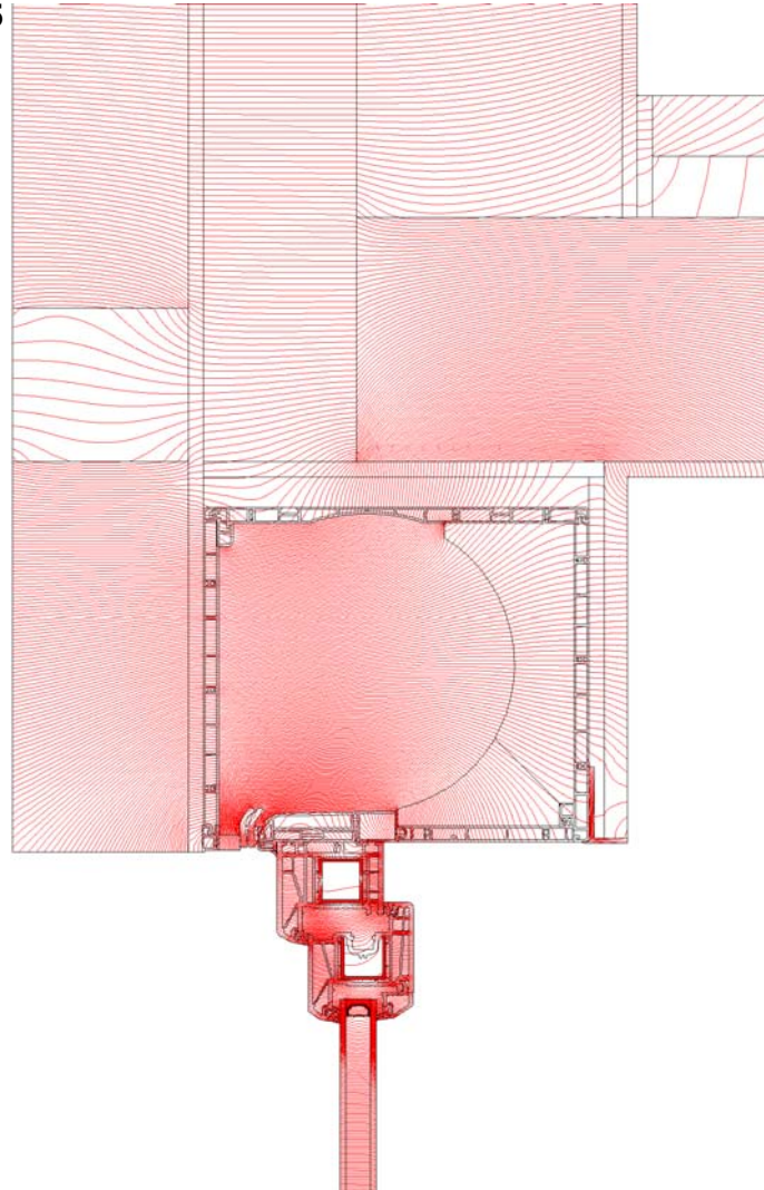
Bild 8 : Einbaudetail
