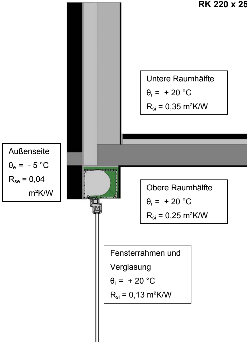
Bild 7 : Einbaudetail mit EXTE Expert RK 220 x 255 Aufbereitung von Bild 1
