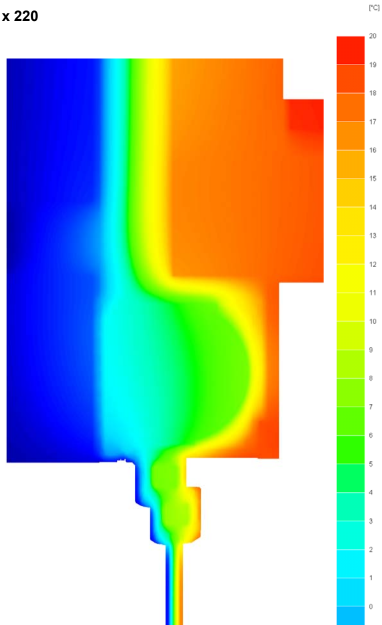
Bild 10 : Einbaudetail mit EXTE Expert RK 220 x 220 (Ausschnitt zur besseren Sichtbarkeit des RK-Bereiches)
