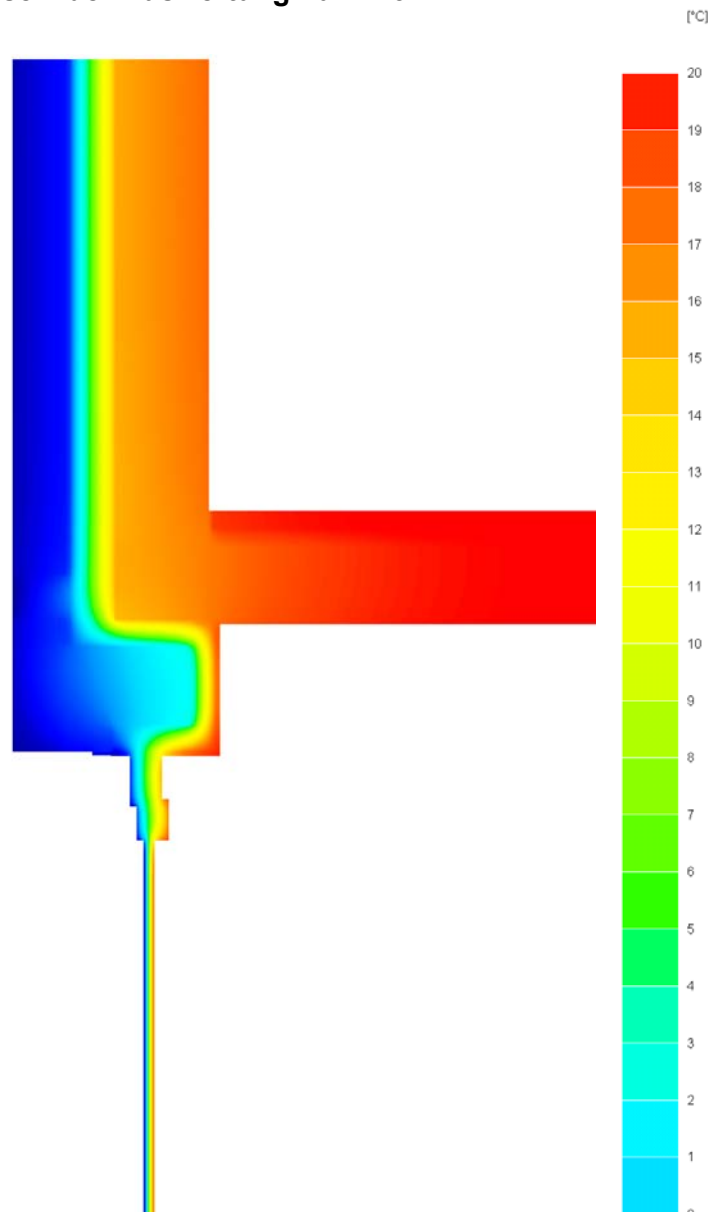
Bild 6 : Einbaudetail B.32
