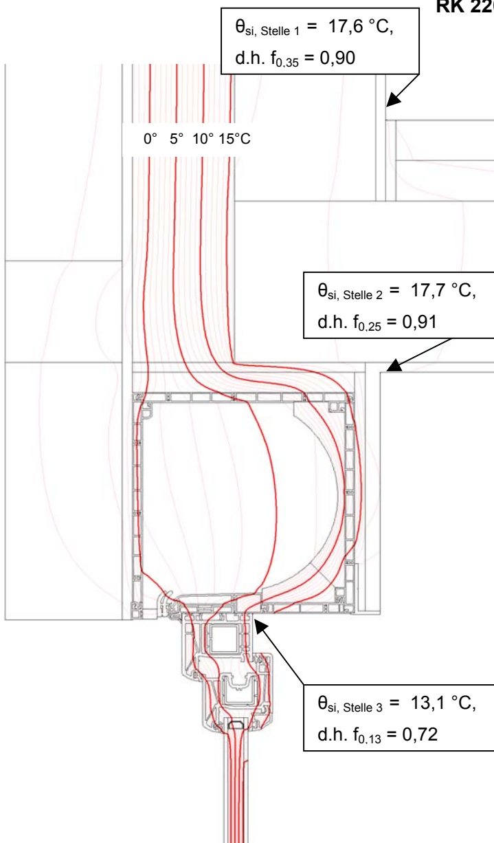
Bild 9 : Einbaudetail mit EXTE Expert RK 220 x 220 (Ausschnitt zur besseren Sichtbarkeit des RK- Bereiches)
