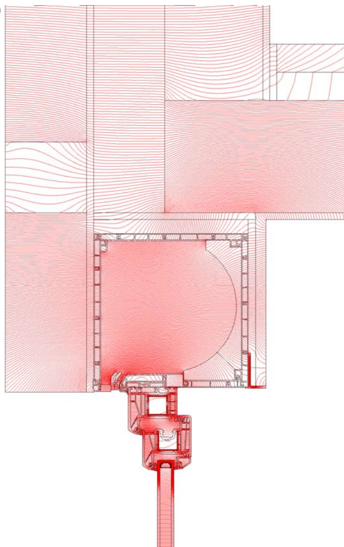
Bild 8 : Einbaudetail
