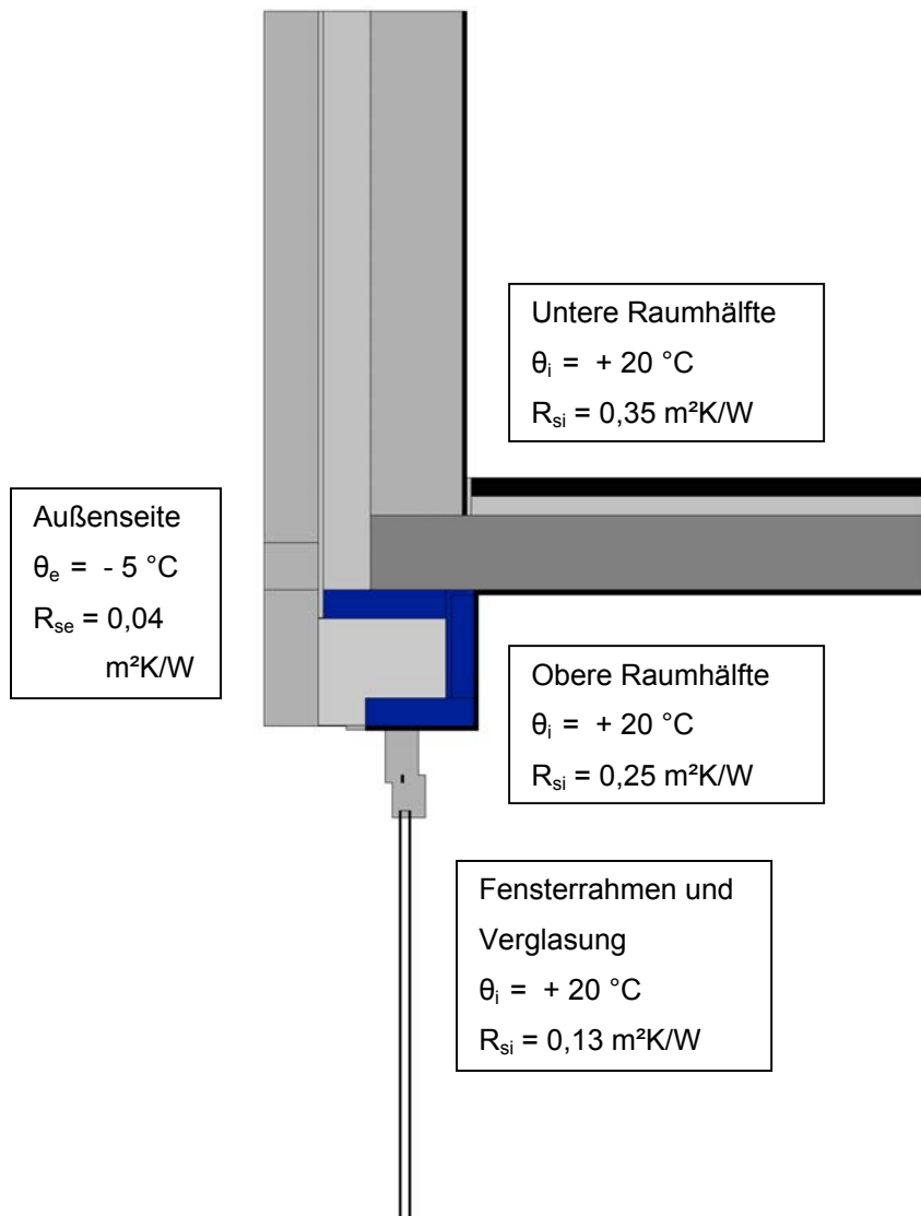
Bild 3 : Einbaudetail B.32
