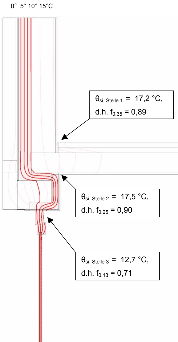
Bild 5 : Einbaudetail B.32
