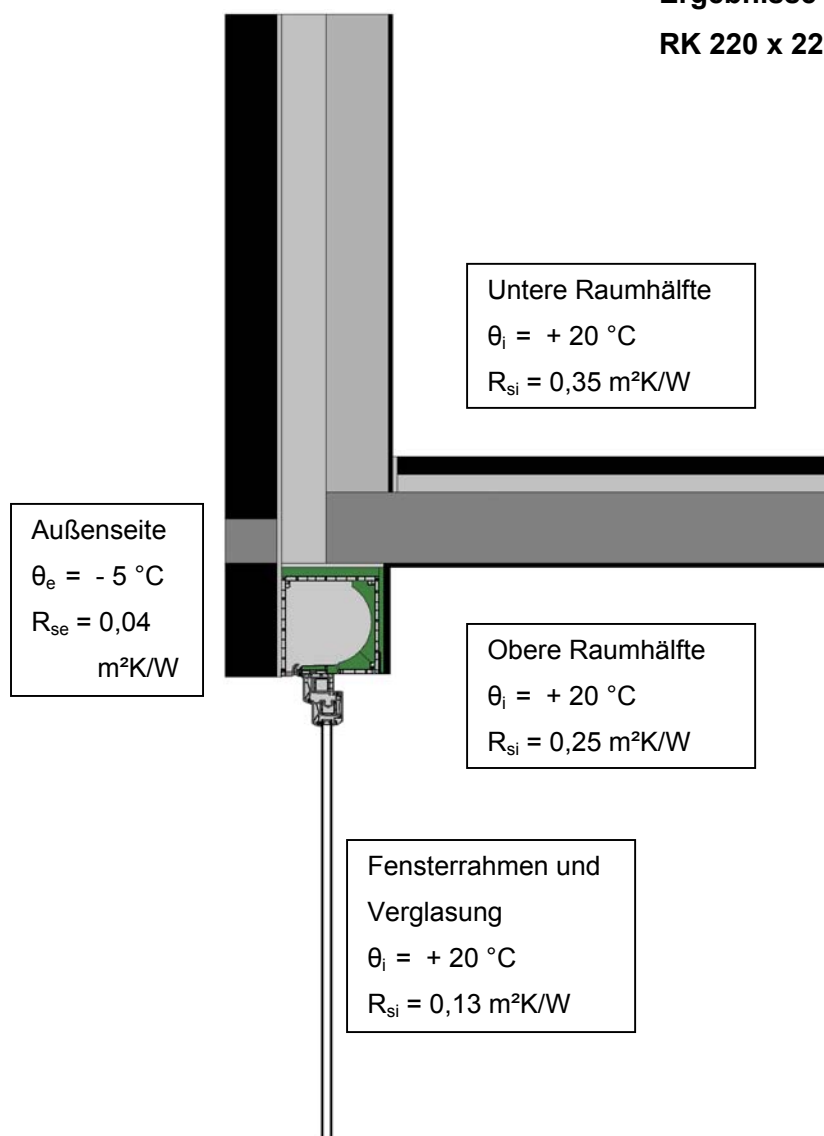
Bild 7 : Einbaudetail mit EXTE Expert RK 220 x 220
